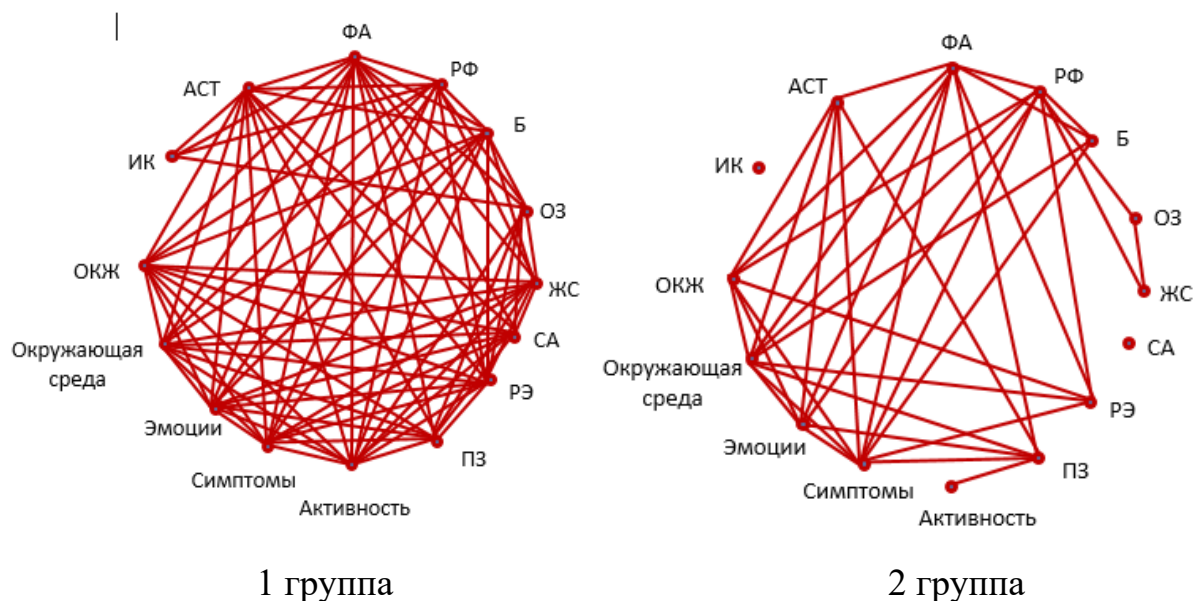
Рисунок 7 – Корреляционные взаимосвязи доменов КЖ по вопросам SF-36 и AQLQ, индекса курения и контроля астмы в когорте городских (1 группа) и сельских жителей (2 группа) 5
