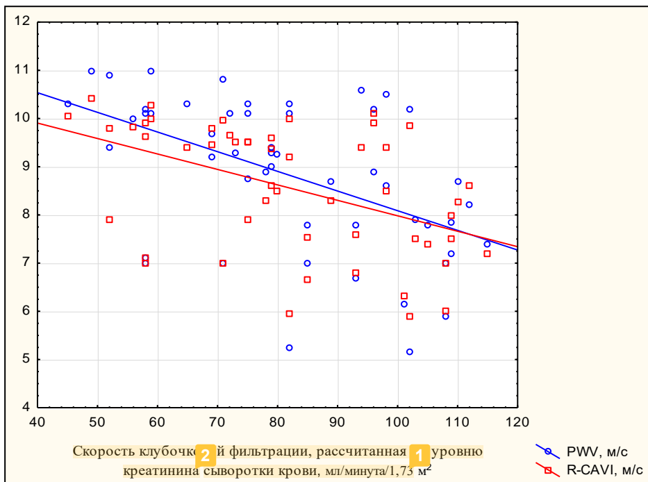
Рисунок 13 – Корреляция между уровнем PWV и СКФ-ЦисСсыв, R-CAVI и СКФ-ЦисСсыв
